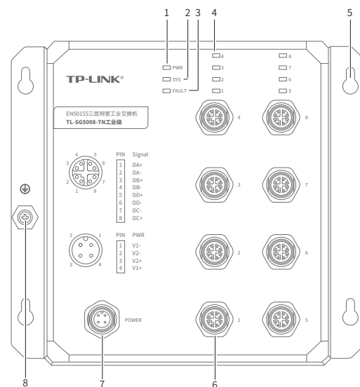
TL-SG5008-TN工业级前面板示意图
